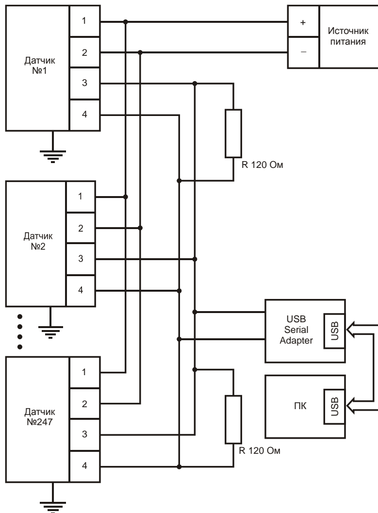
Рис. 3 Схема подключения датчиков КОРУНД-ДИ-001MRS-552 в групповом режиме
