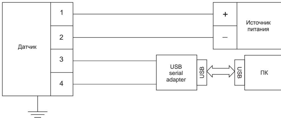
Рис. 2 Схема подключения датчиков КОРУНД-ДИ-001MRS-552 в монорежиме
