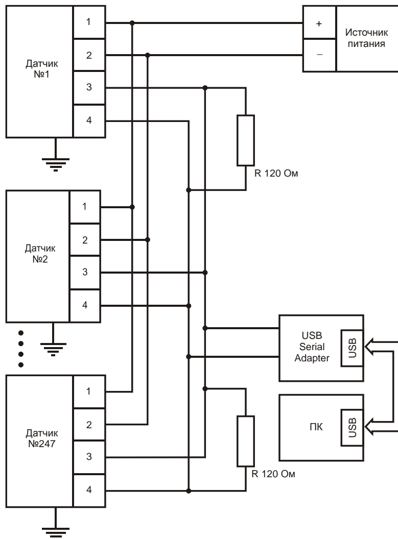
Рис. 3 Схема подключения датчиков КОРУНД-ДИ-001MRS-558 в групповом режиме
