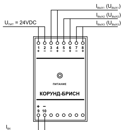
Подключение двухпроводных датчиков
