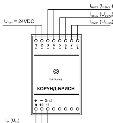
Подключение трехпроводных датчиков
