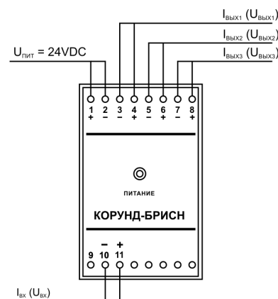
Подключение активных источников сигналов
